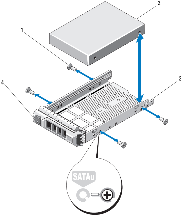
그림 16-5. 3.5" 하드 드라이브 캐리어에 하드 드라이브 분리 및 설치
