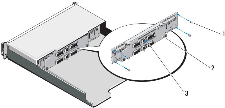
그림 16-17. 후면판 -PowerVault MD3620i 분리 및 설치
