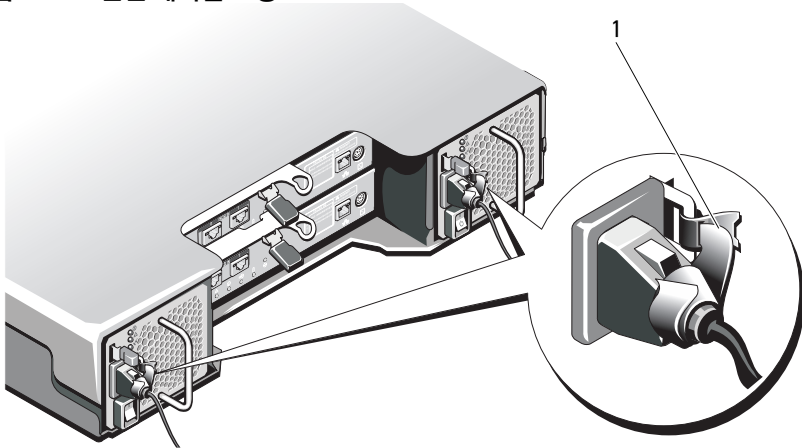
그림 16-12. 전원 케이블 고정
