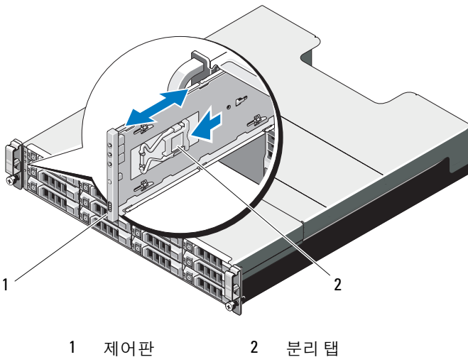
그림 16-13. 제어판 -PowerVault MD3600i 분리 및 설치
