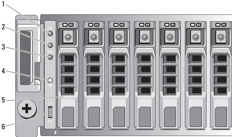
그림 2-2. 전면 패널 기능 및 표시등 — Dell PowerVault MD3620i
