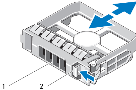
그림 16-2. 3.5" 하드 드라이브 보호물 분리 및 설치 (MD3600i 에만 해당됨 )
