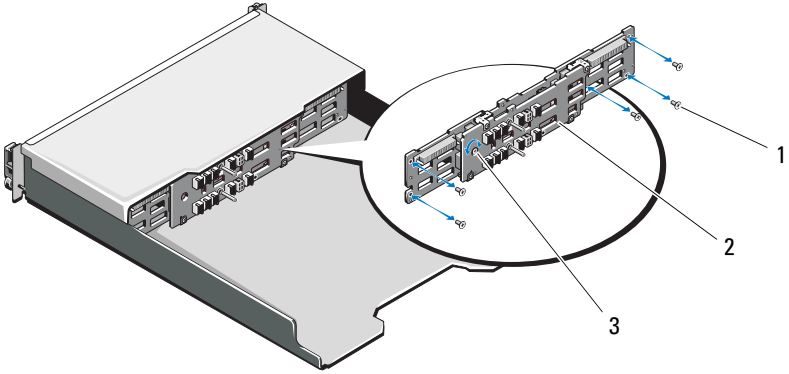
그림 16-16. 후면판 -PowerVault MD3600i 분리 및 설치
