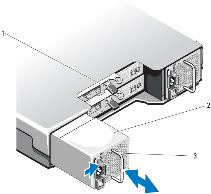
그림 16-11. 전원 공급 장치 / 냉각팬 모듈 분리 및 설치
