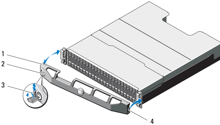
그림 16-1. 전면 베젤 분리 및 설치
