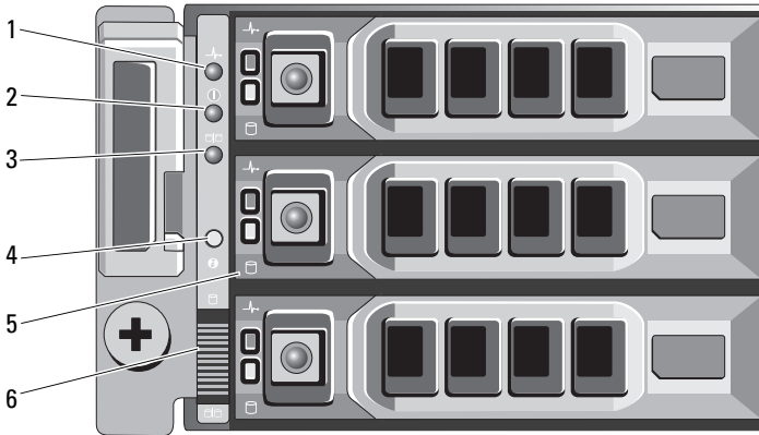
그림 2-1. 전면 패널 기능 및 표시등 — Dell PowerVault MD3600i
