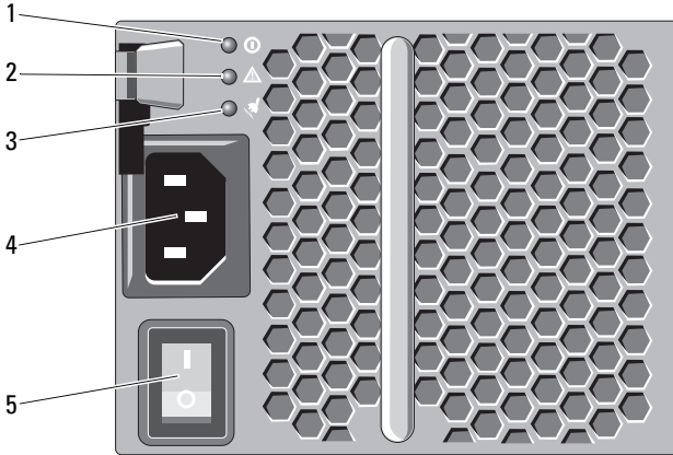
그림 2-6. 전원 표시등 코드 및 기능
