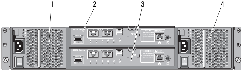
그림 2-4. 후면 패널 기능 및 표시등 — Dell PowerVault MD3600i 시리즈 스토리지 배열
