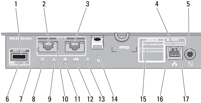
그림 3-1. MD3600i 시리즈 iSCSI RAID 컨트롤러 모듈
