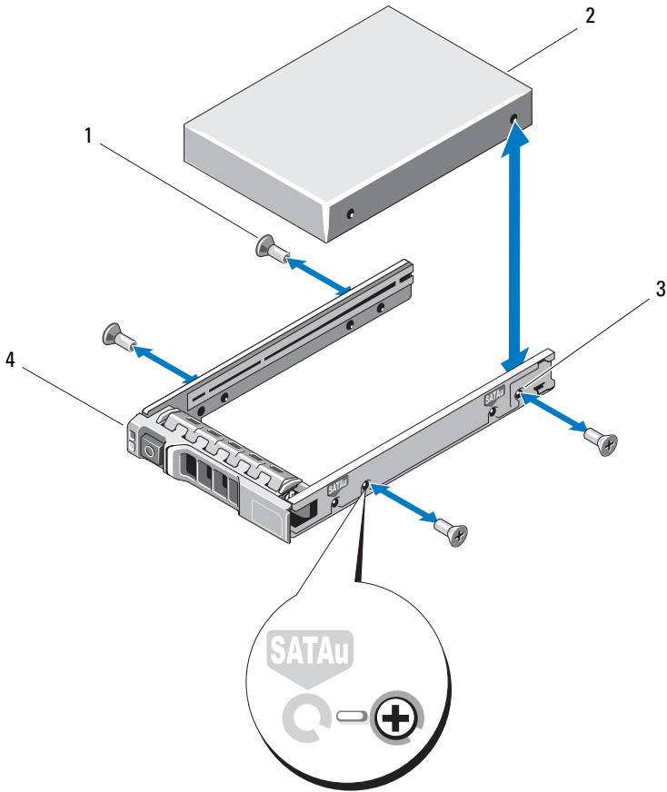
그림 16-6. 2.5" 하드 드라이브 캐리어에 하드 드라이브 분리 및 설치
